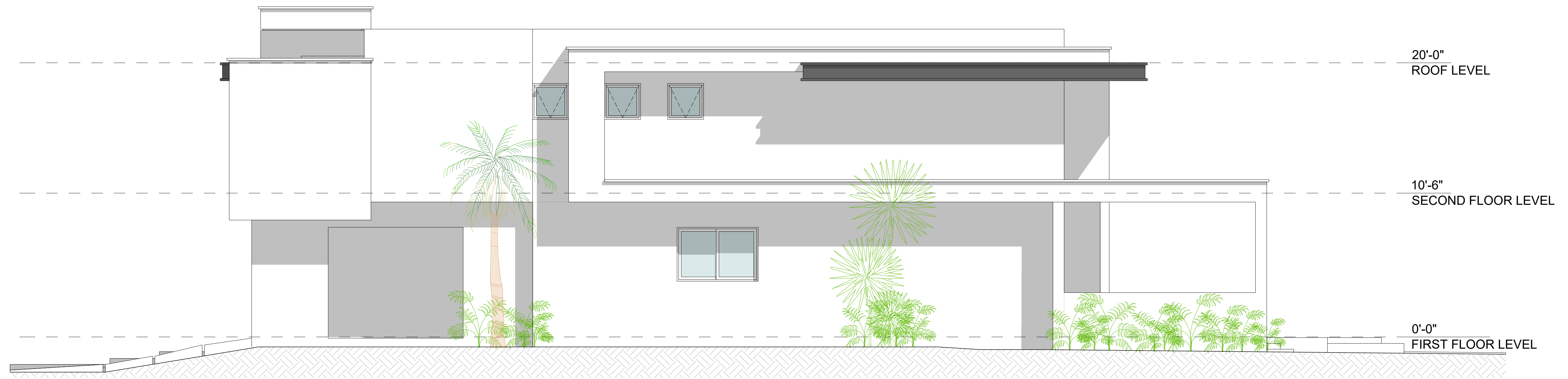
01 RIGHT ELEVATION
