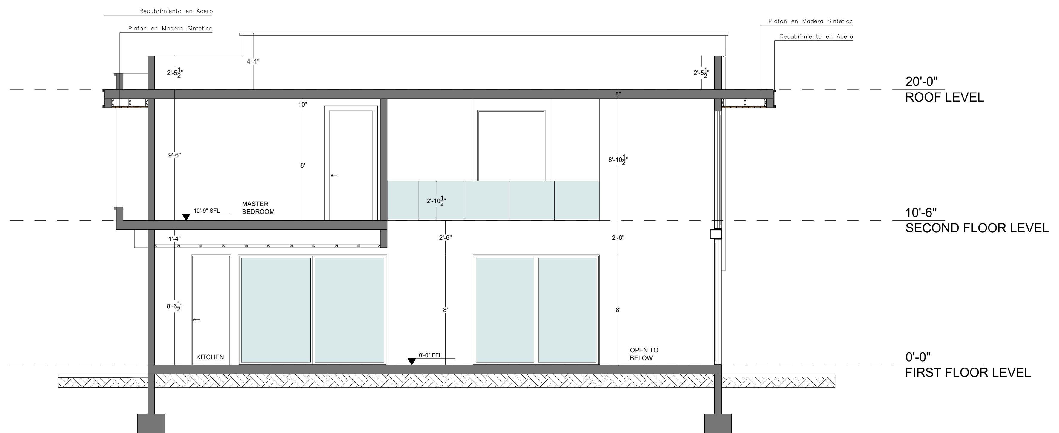
01 SECTION D - D
